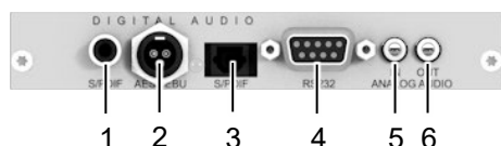
Fig. 23 Interface side L-/R474-BDA
