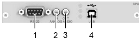
Fig. 12 Interface side L-/R474-BAE/-BRE
